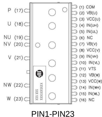
SOP23-FP
