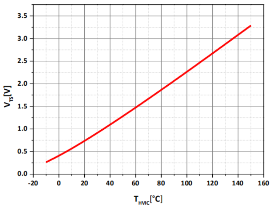
图 5: HVIC 温度检测输出温度—电压曲线
